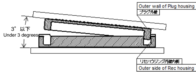
△ 図-2 外壁合せによる嵌合 (Acceptable) Figure-2 Mating aligning to outer wall of housings (Acceptable)
