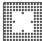
FIG. 346 MHAX-124-X-13B MPAX-124-X-13B
